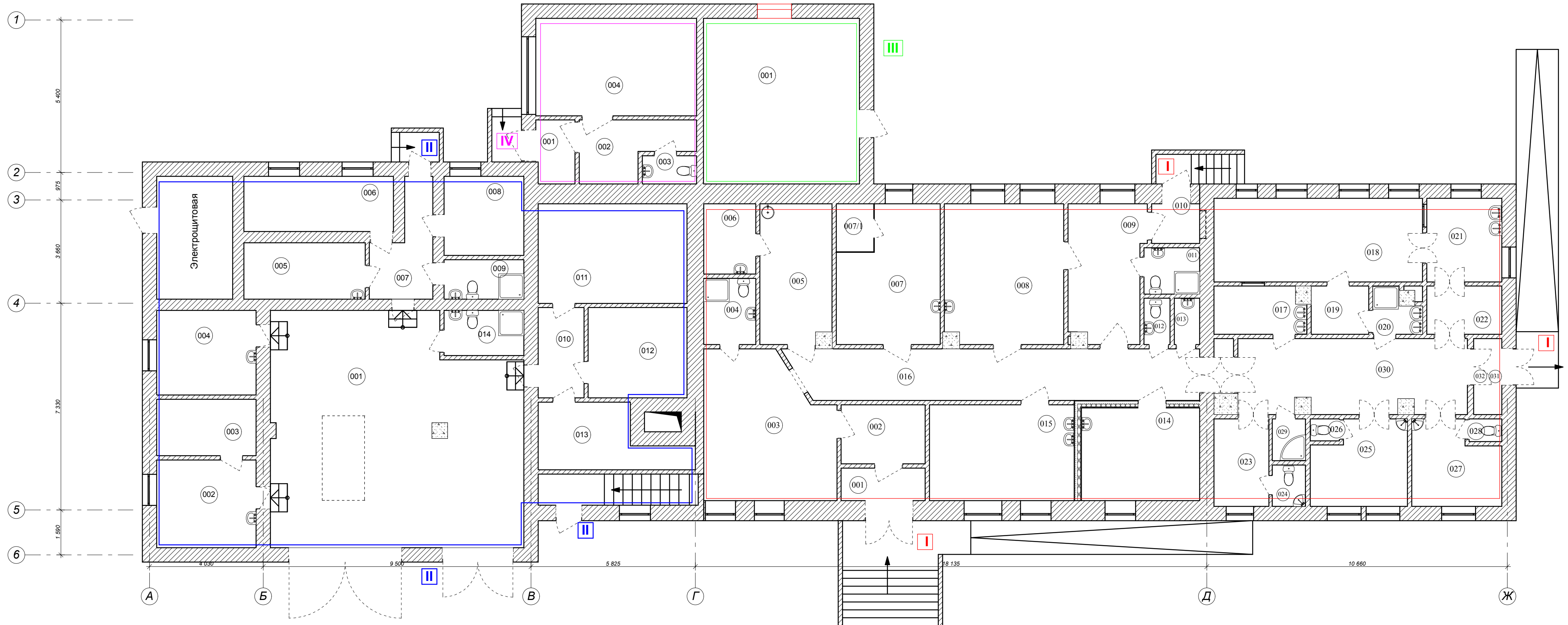
Экспликация помещений стационара №I
