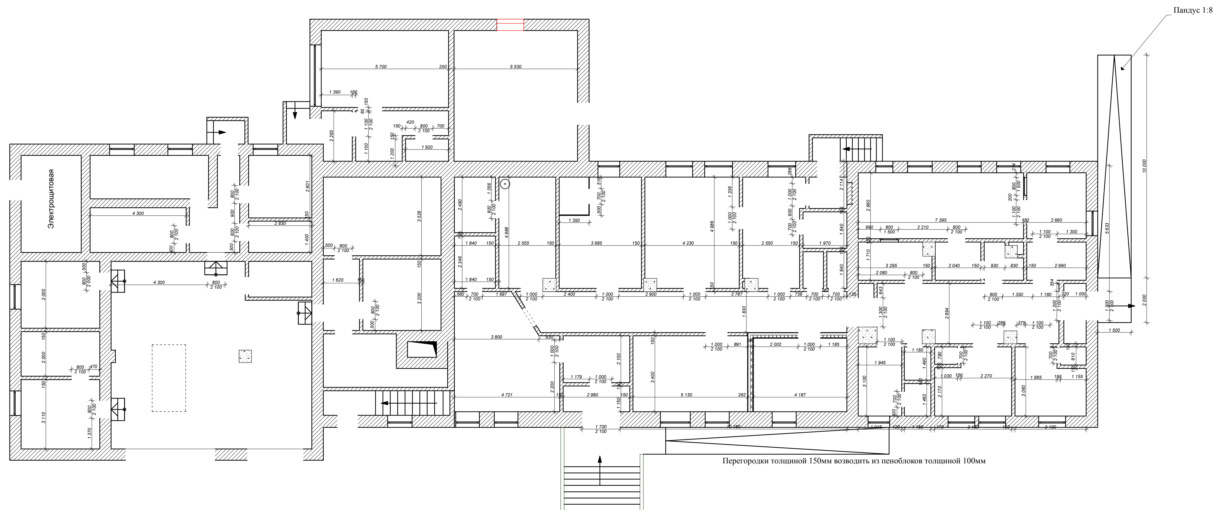
План монтируемых перегородок
